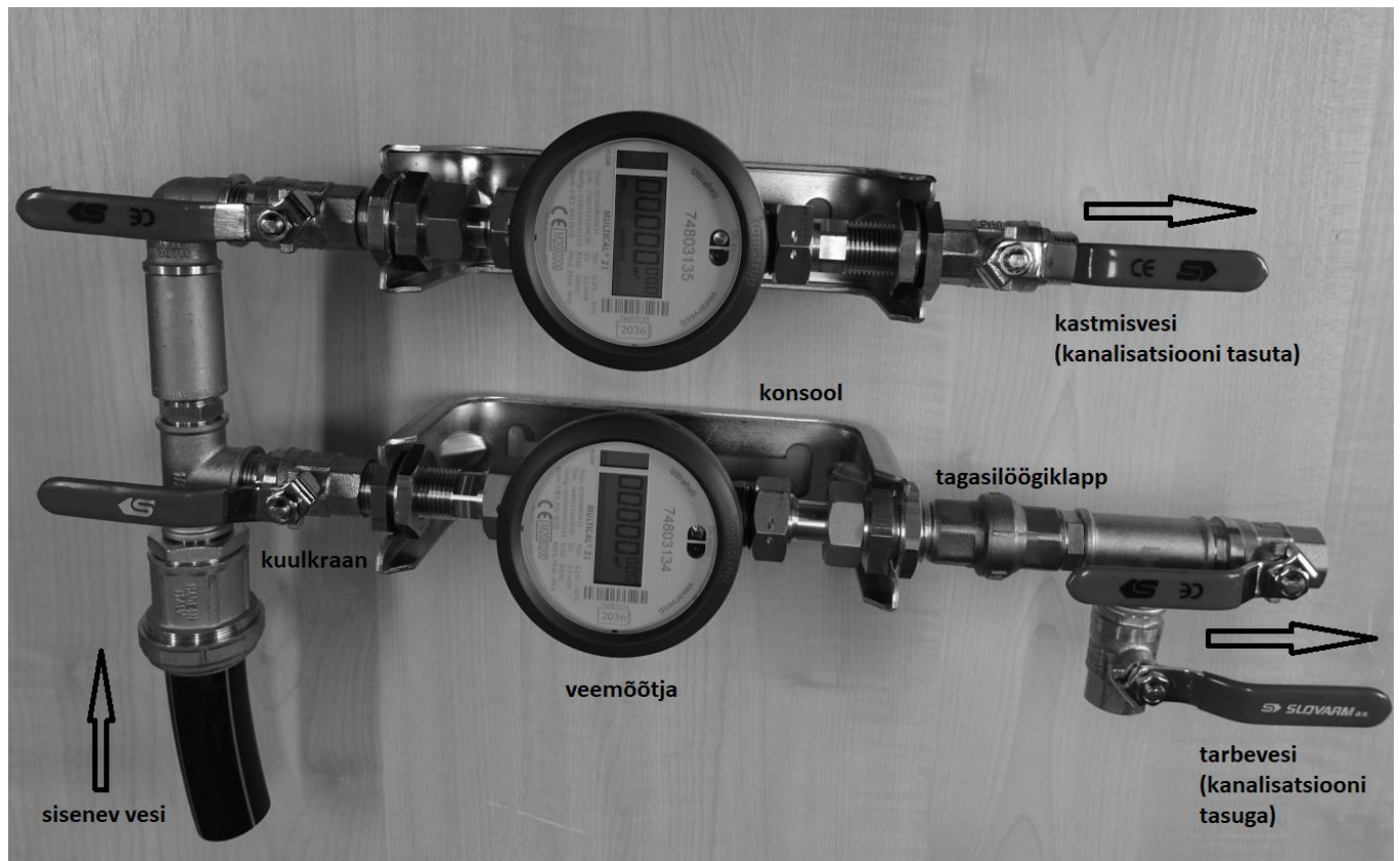
Joonis 1. Kastmisvee ja tarbevee mõõtesõlm.
