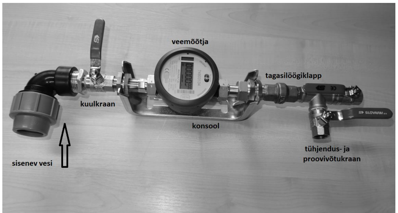
Joonis 2. Tarbevee mõõtesõlm.
